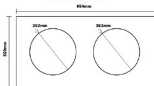
Reforço do painel frontal ou baffle
